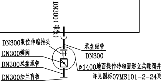
J9-1、J9-2、J13-1、J32-2、J38-1、J44-1、 J49-1、J50-1、J52-1、J64-1、J64-2 阀门节点（一） 共11个
