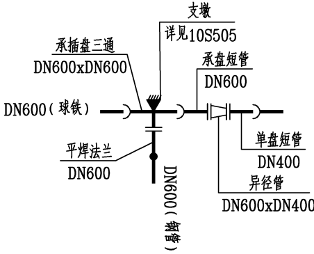
J29 三通节点（八） 共1个
