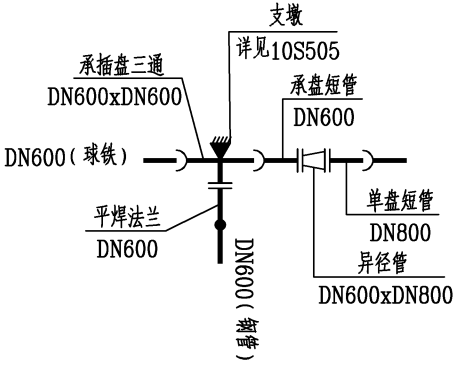
J27 三通节点（七） 共1个
