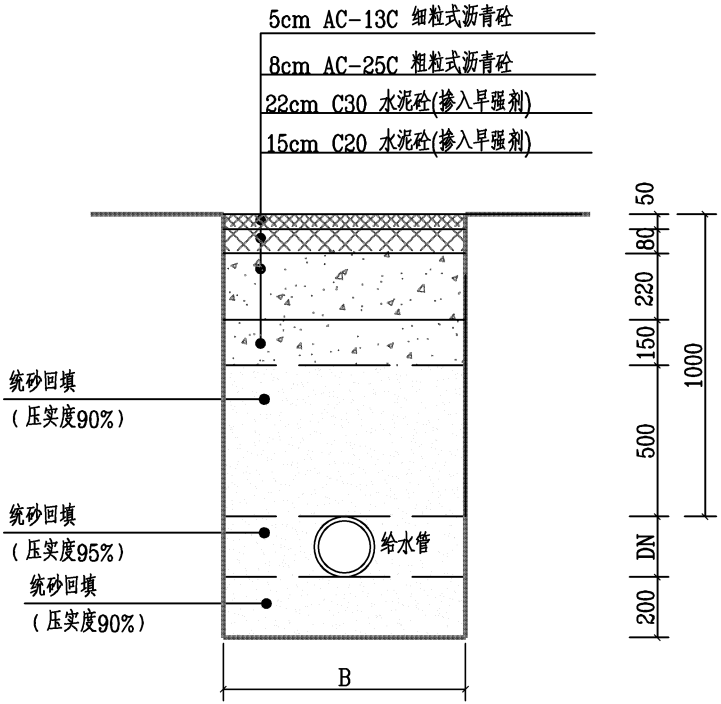
沥青路面管沟开挖回填断面图
