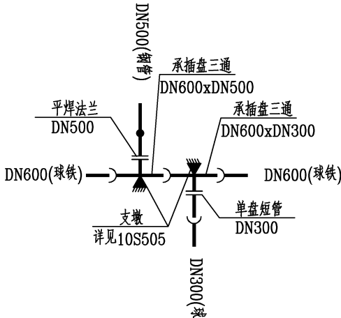
J32 三通节点（六） 共1个
