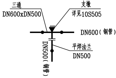
J23、J32 三通节点（四） 共2个
