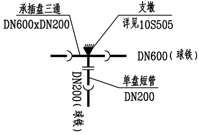
J36、J39 三通节点（三） 共2个
