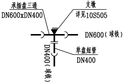
J4 三通节点（一）
