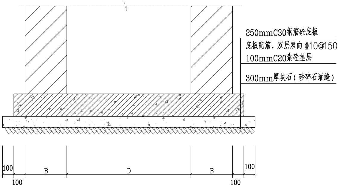
井基础处理示意图
