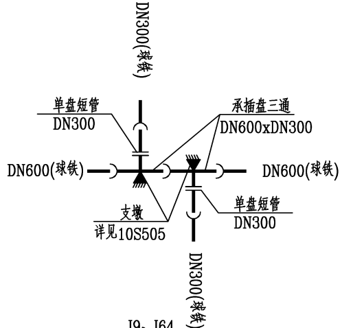
J9、J64 三通节点（五） 共2个
