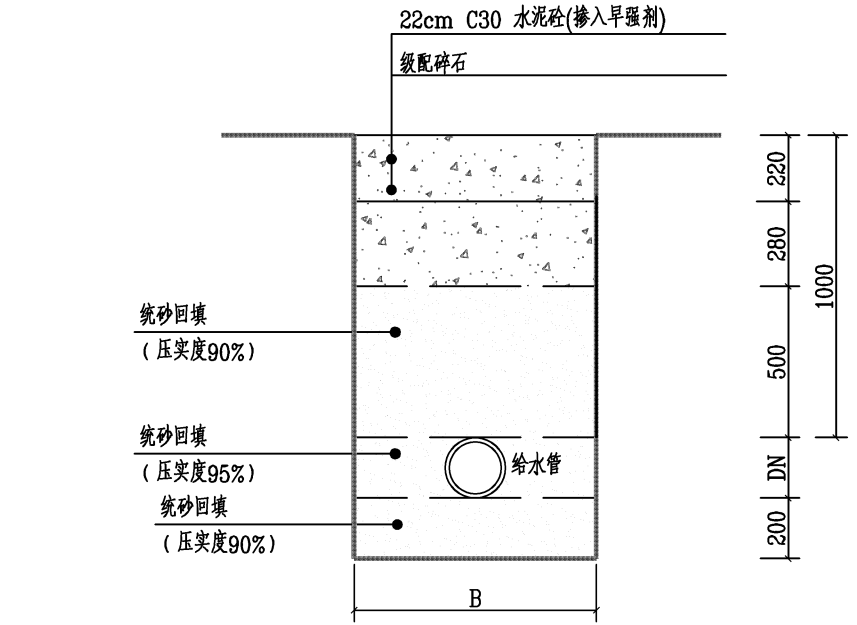
砼路面管沟开挖回填断面图
