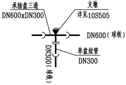
J9、J32、J38、J44、J49、J50、J52、J64 三通节点（二） 共8个
