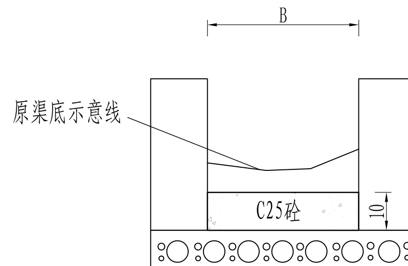
整修渠道标准横断面图(二) 1:10 渠底清淤+渠道底板
