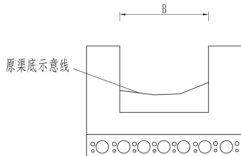
整修渠道标准横断面图(一) 1:10 渠底清淤
