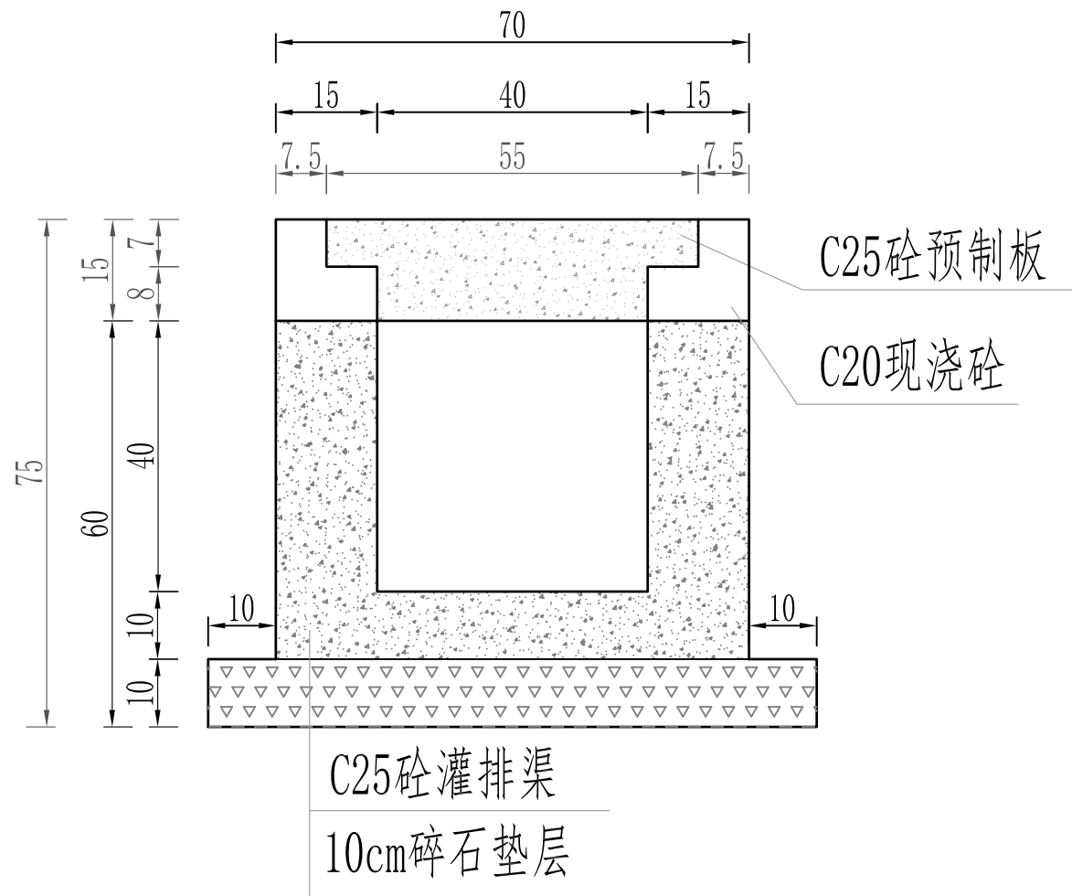
新建40×40cm灌排渠预制盖板断面图
