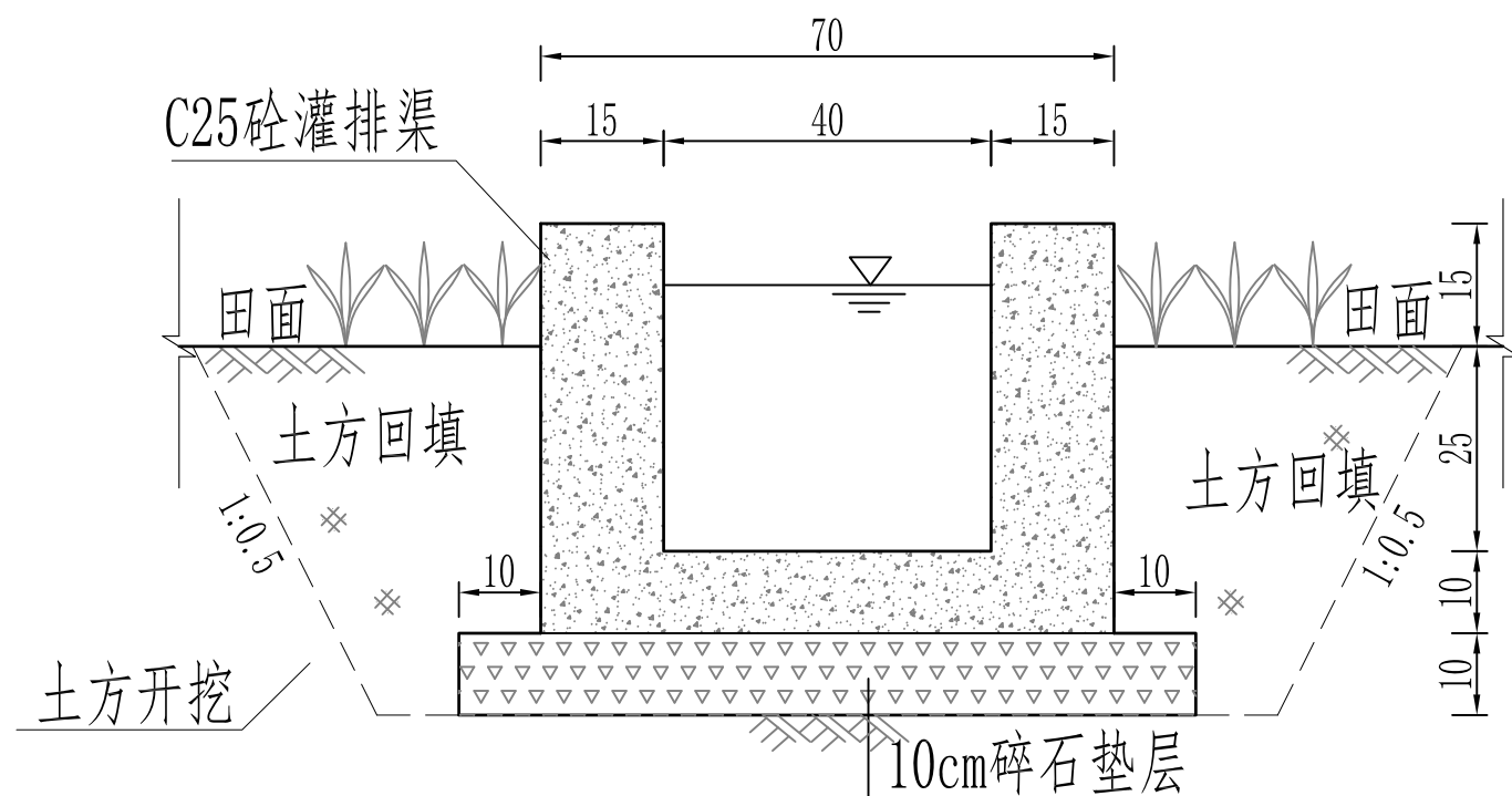
新建40×40cm灌排渠断面图 1:10
