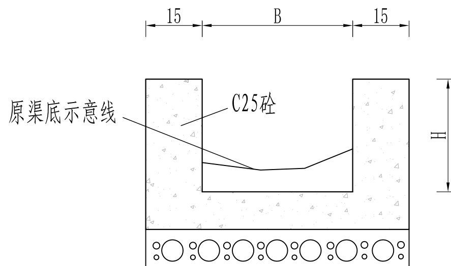
整修渠道标准横断面图(四) 1:10 渠道一段修补(含侧墙、底板)
